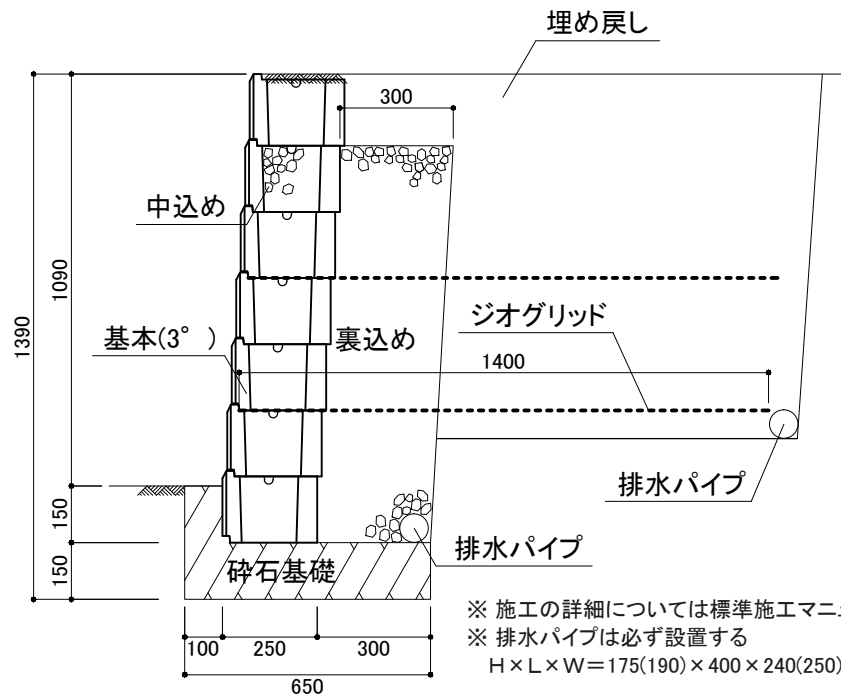
ABロック3° 7段積(1090)
